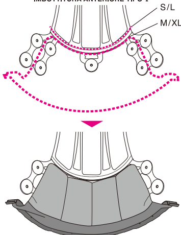
VORDERES POLSTER TYP-I IMBOTTITURA ANTERIORE TIPO-I
